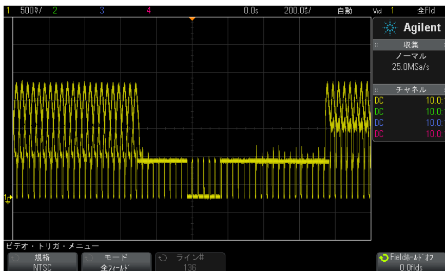
図 18 すべてのフィールドでのトリガ
