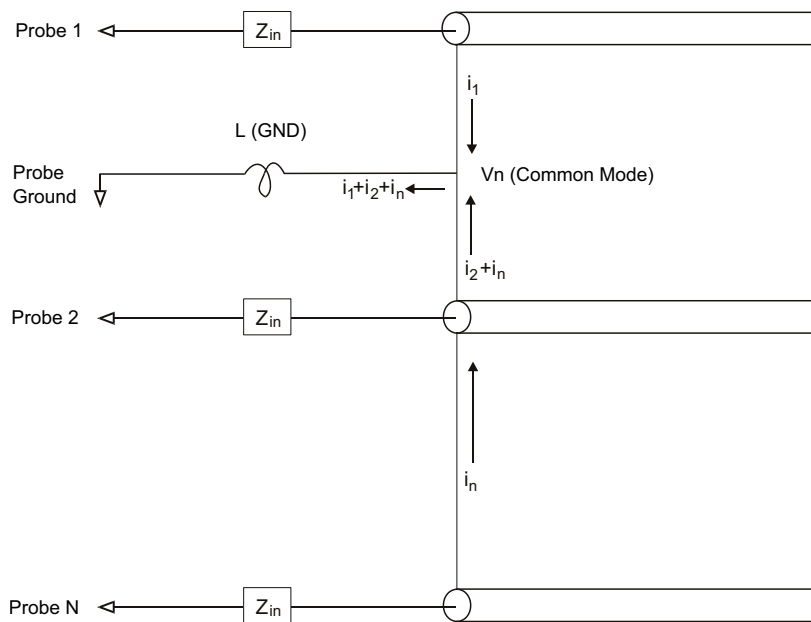
図 12 コモン・モード入力電圧モデル
