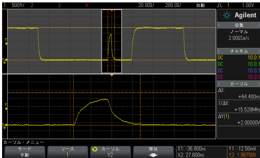
図 30 カーソルによるズーム・ウィンドウのトラッキング
