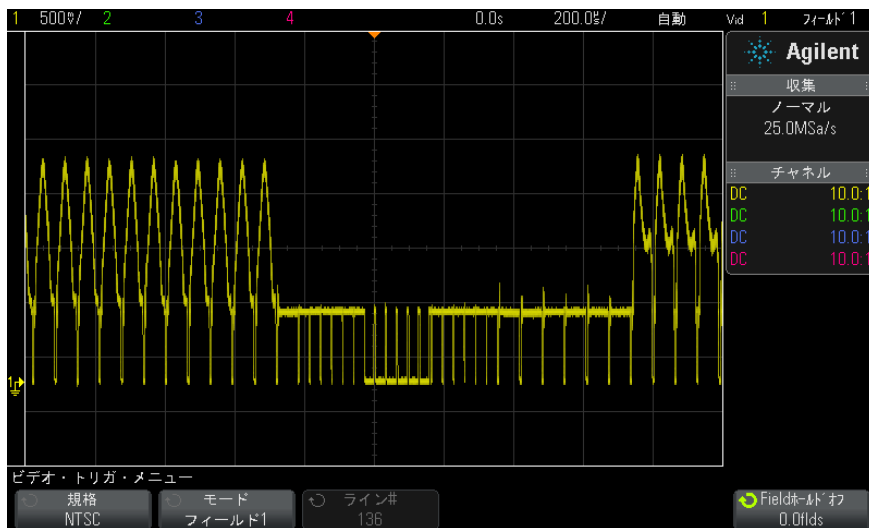
図 17 フィールド1でのトリガ
