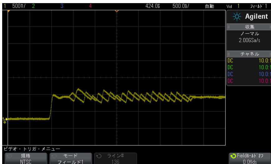
図 19 カラー・フィールド1とカラー・フィールド3での交互のトリガ
