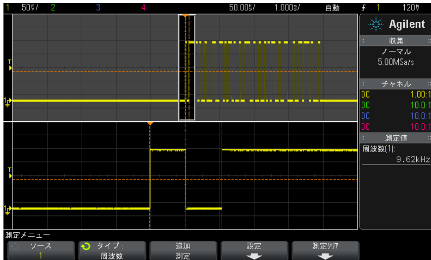
図 35 周波数測定のエッジの分離
