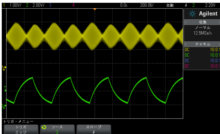
図 14 40 %輝度で表示した振幅変調
