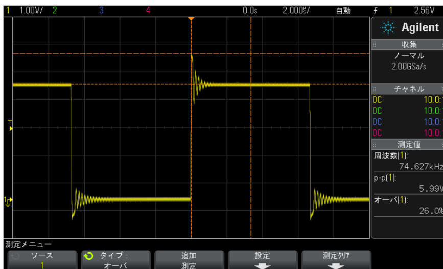
図 34 自動オーバシュート測定
