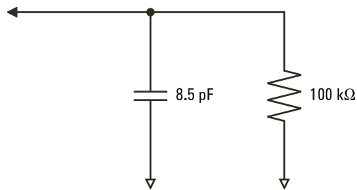
図 9 DC および低周波プローブ等価回路
