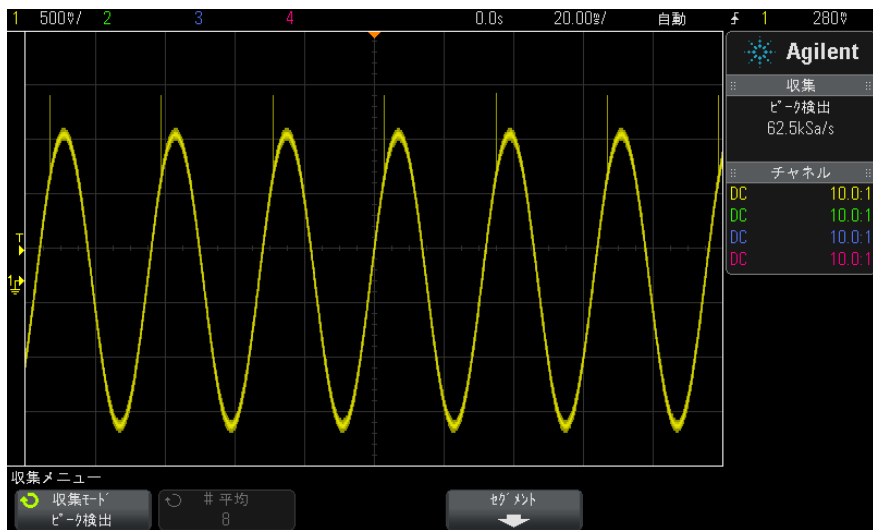
図 25 グリッチのある正弦波、ピーク検出モード
