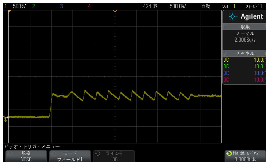
図 20 フィールド・ホールドオフを使ったカラー・フィールド1または3との同期（フィールド1モード）
