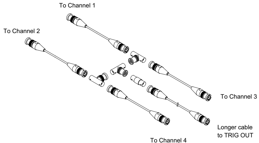
図 37 4チャンネル・オシロスコープ用のユーザ校正ケーブル
