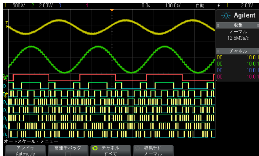
図 8 例：デジタル・チャンネルのオートスケール（MS0 モデルのみ）
