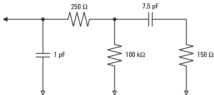
図 10 高周波プローブ等価回路
